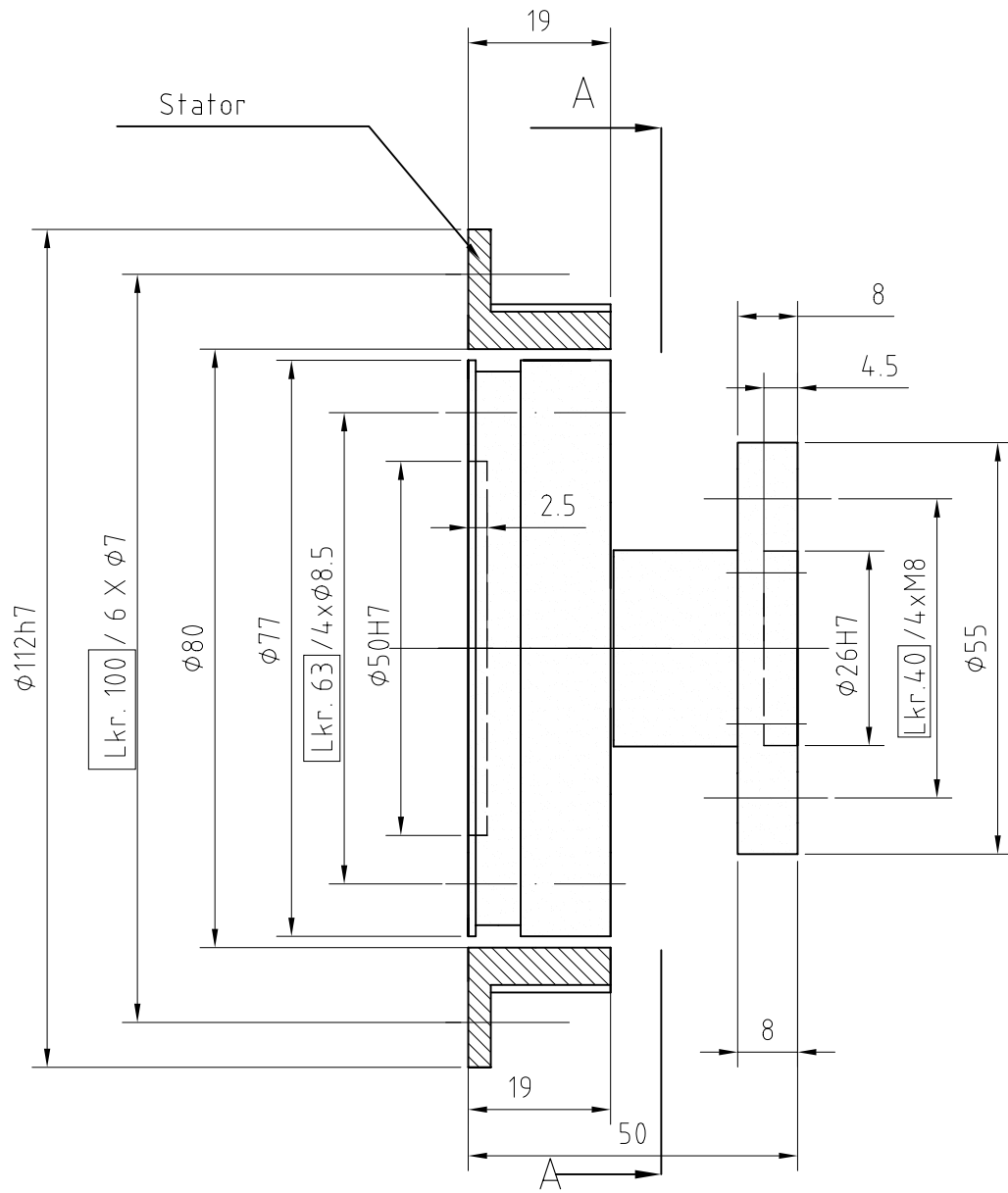
Ansicht B - B
